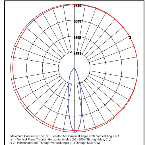
WCTRSDC31X20U41K 30° Reflector
